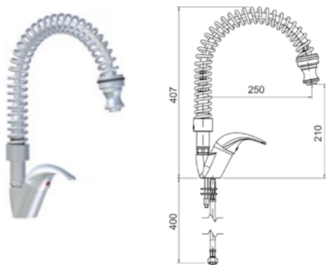
Modelo Código Grifo mezclador monomando espiral • R0020239
