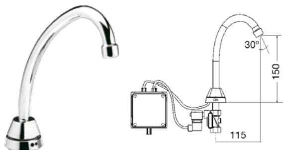
Modelo Código Grifo electrónico de caño alto a red • R0020230
