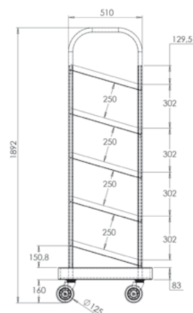
MEDIDAS CARRO
