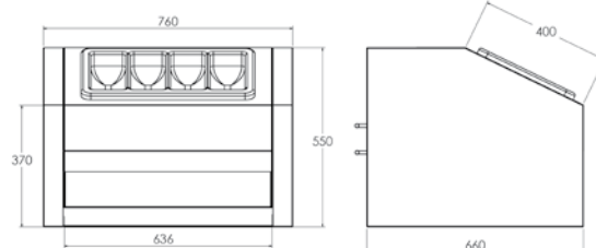
MEDIDAS DISPENSADOR
