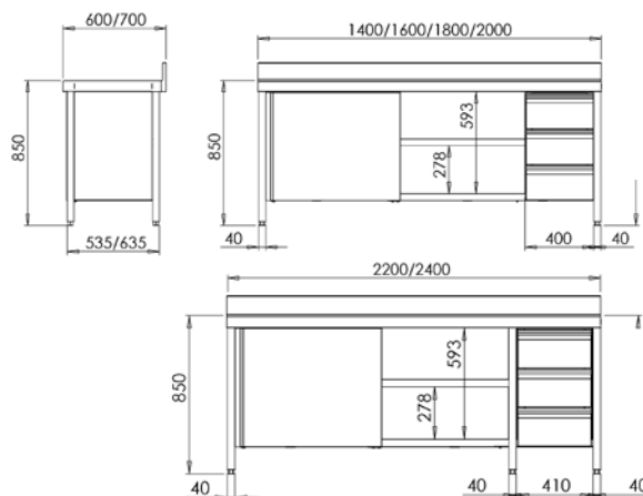
MEDIDAS MESA MURAL CON PUERTAS Y CAJONES
