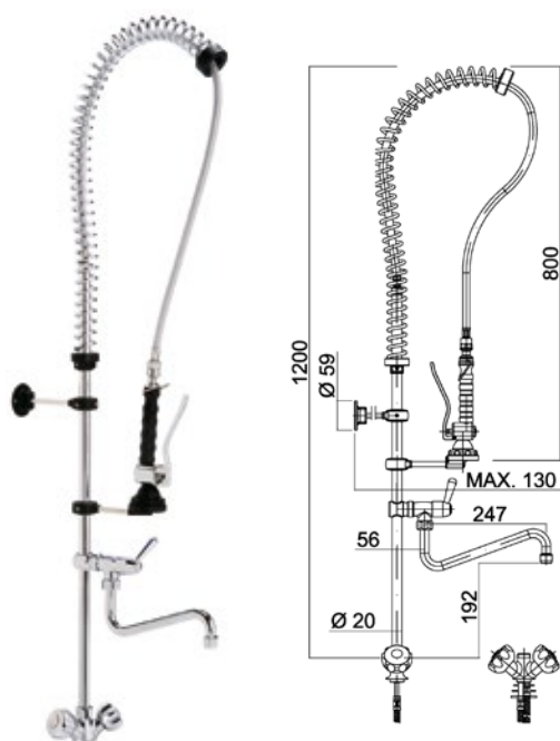
Modelo Código Grifo ducha dos aguas con grifo • R0020301
