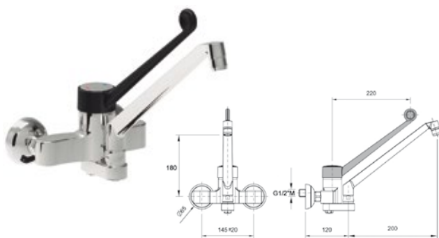
Modelo Código Grifo mezclador de pared dos aguas • R0020222
